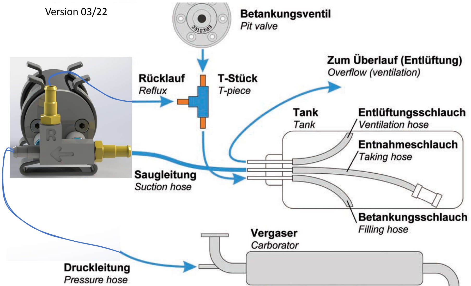
Abbildung 1: Anschlussschema picture 1: connection scheme
